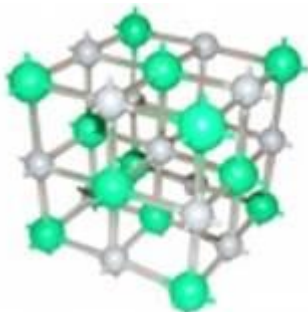
Рис. 2. Пример кристаллической решётки (каменная соль)
