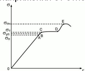
Рис. 4. Диаграмма растяжений
